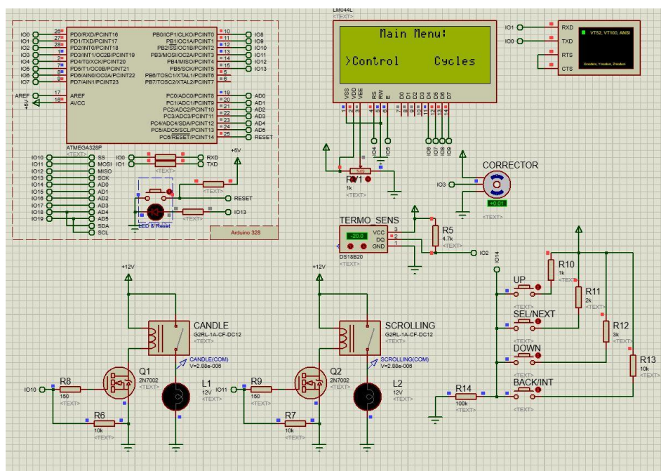
Рисунок 2 – Моделирование в программе Proteus
