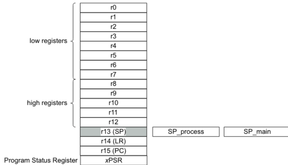
Рисунок 1 – Регистры arm-m3/m4-процессора
