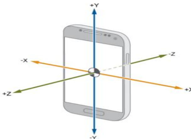
Рисунок 1 – Пример датчика акселерометра
